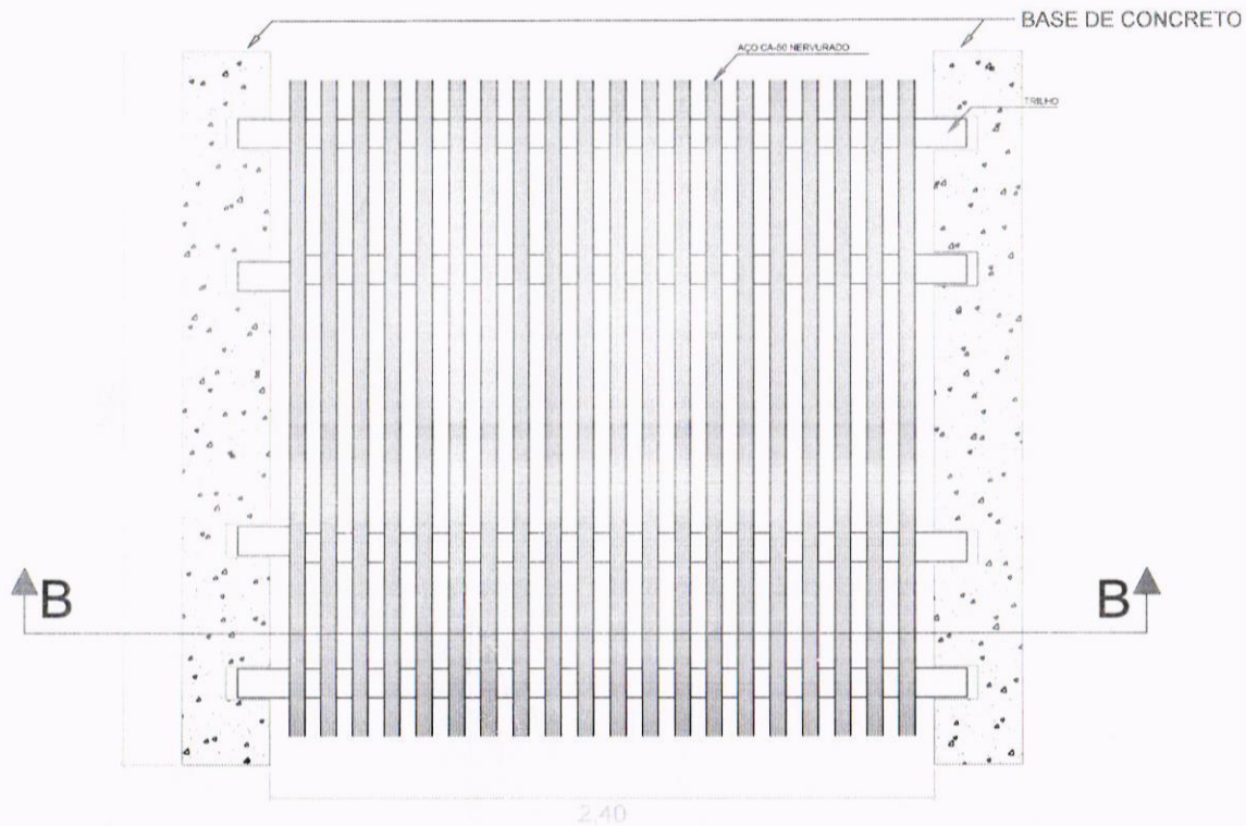
PLANTA BAIXA MATA BURRO
