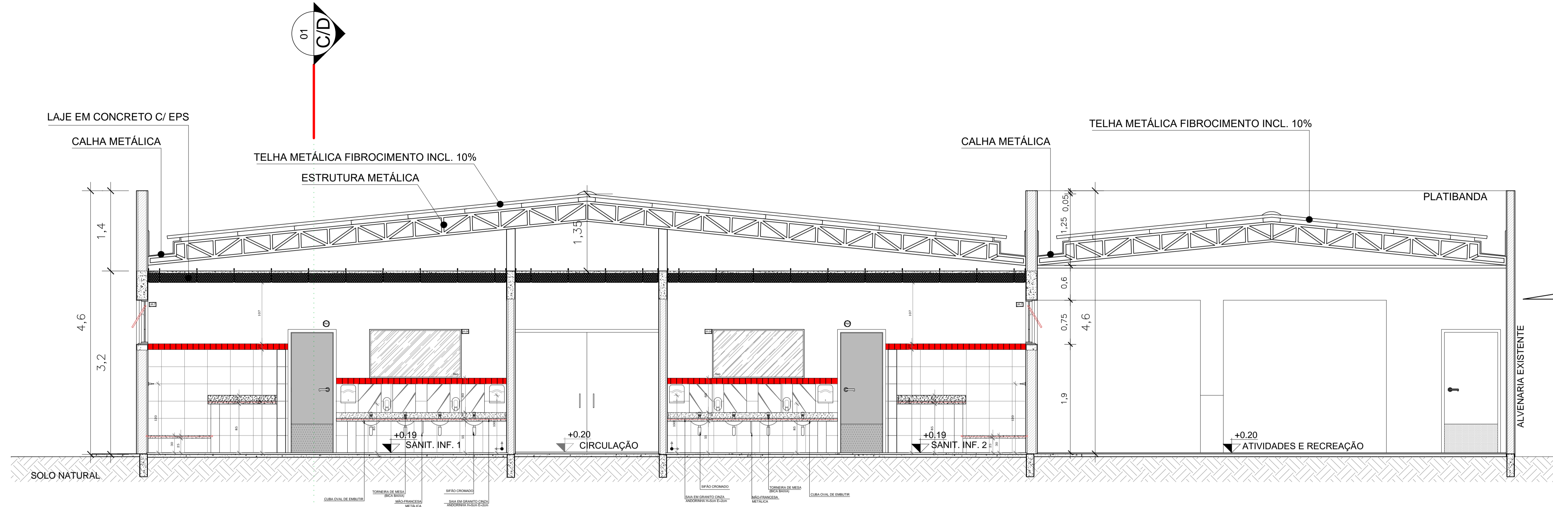
02 CORTE A-B ESCALA 1/40
