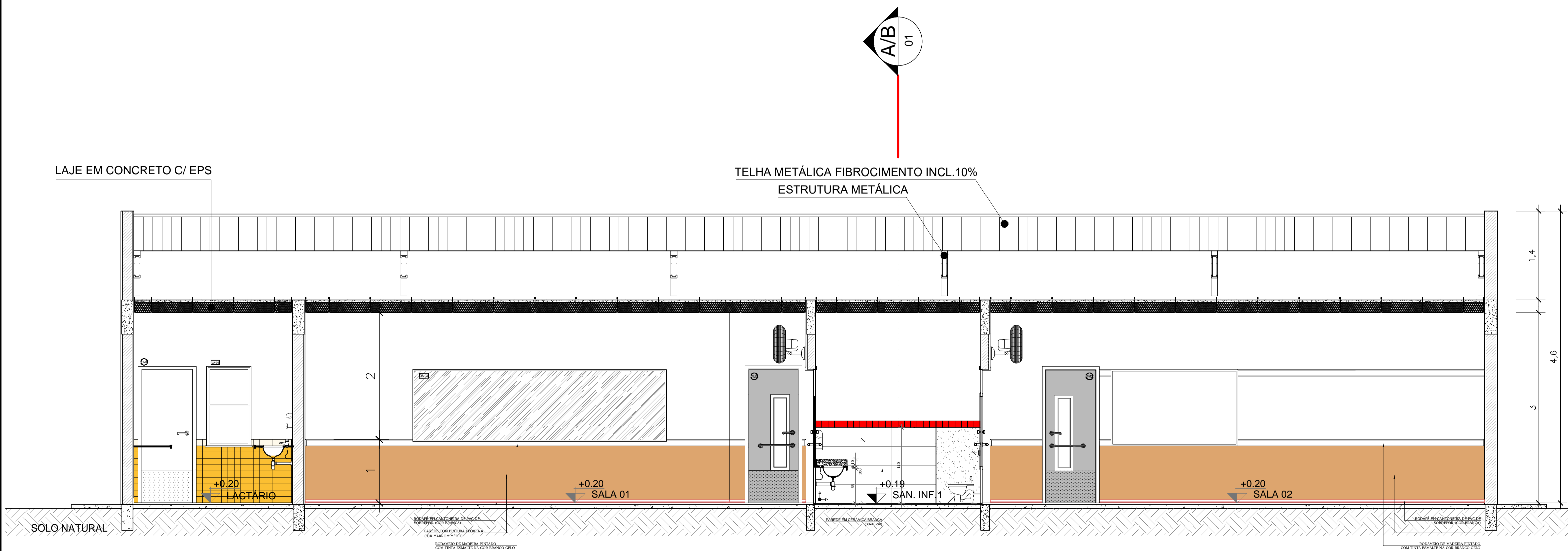
01 CORTE C-D ESCALA 1/50
