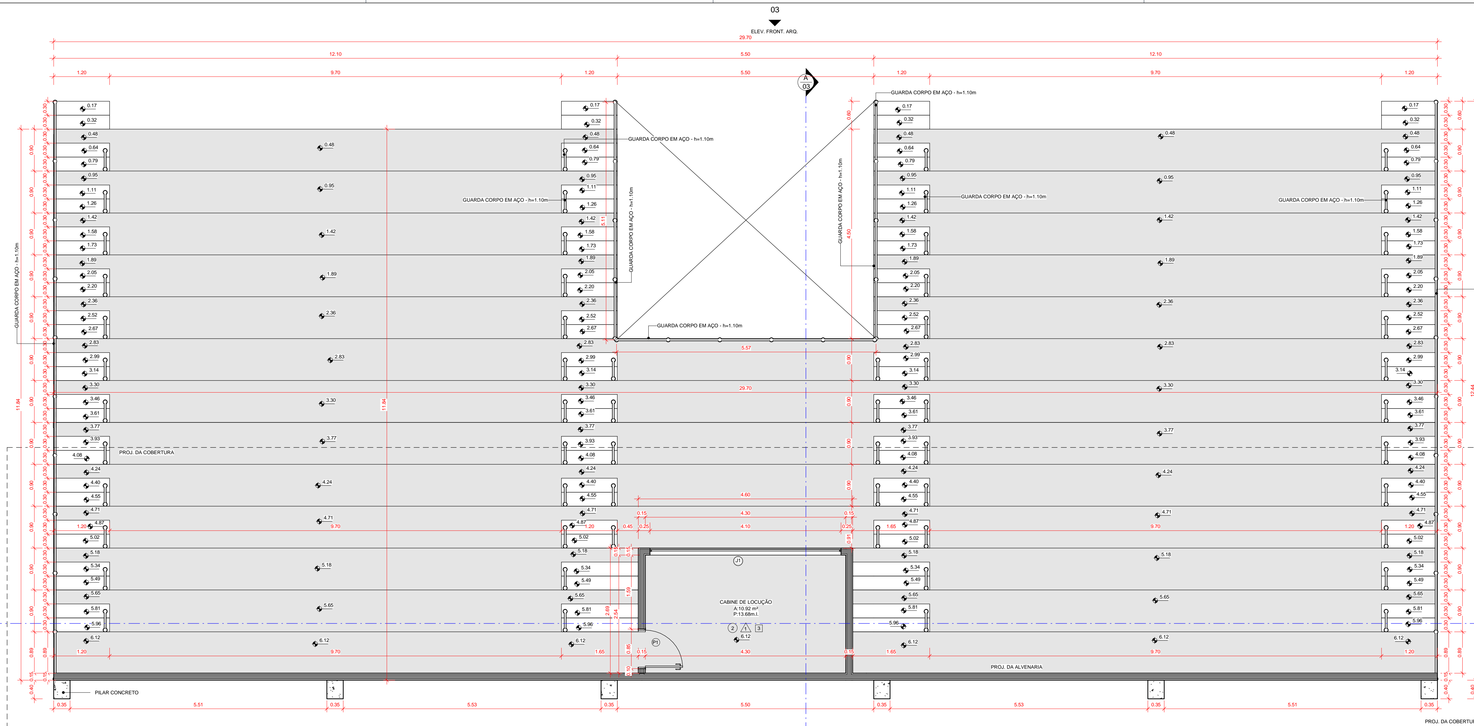
2 PLANTA BAIXA - ARQUIBANCADAS 1: 50
