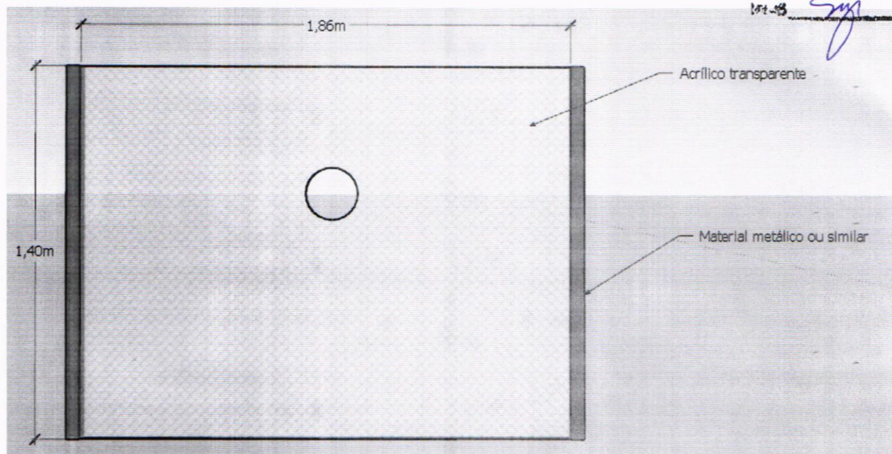
Figura 02 – Painel nº 02 – Dimensões e especificações
