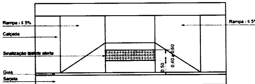
Figura 23 – Rebaixamento de calçada com rampas complementares \le 5\%
