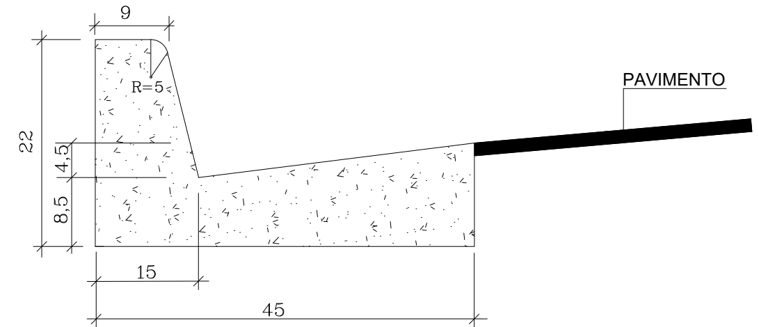
DETALHE DO MEIO FIO E SARJETA SEM ESCALA
